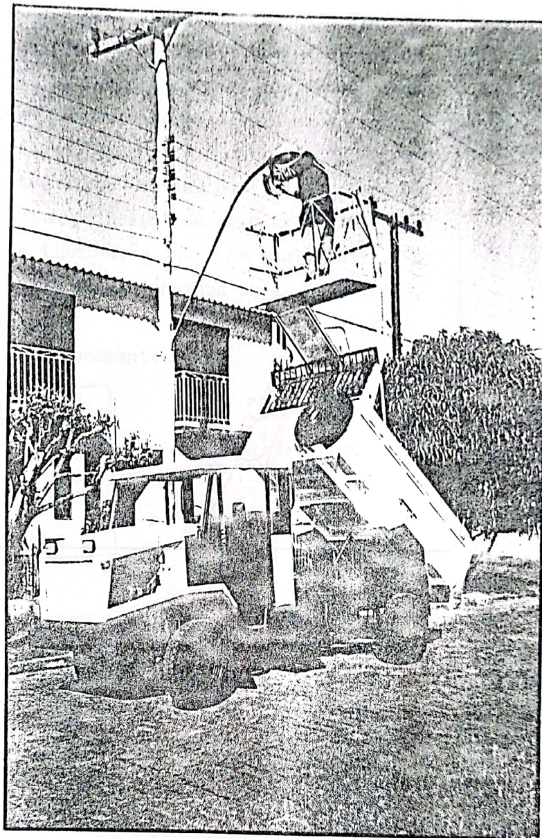
CTT - 1600 B - equipado com plataforma aérea
